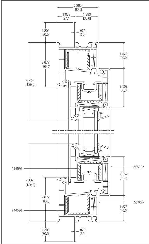
SECTION A-A
