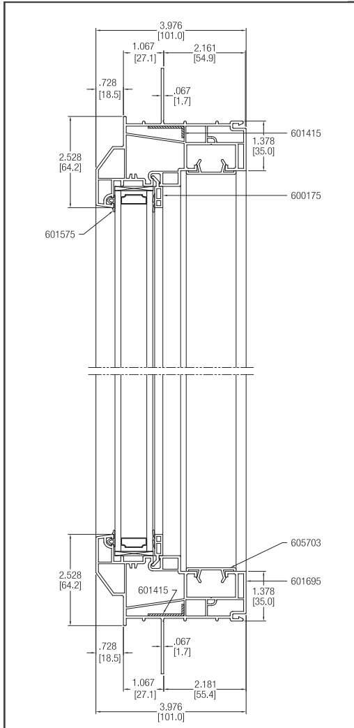
SECTION A-A
