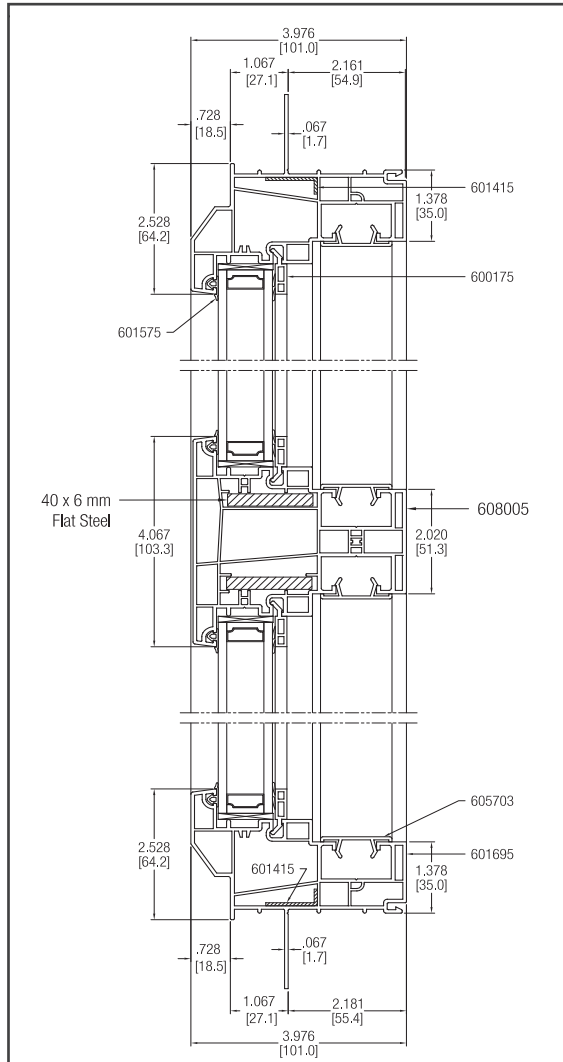
SECTION A-A
